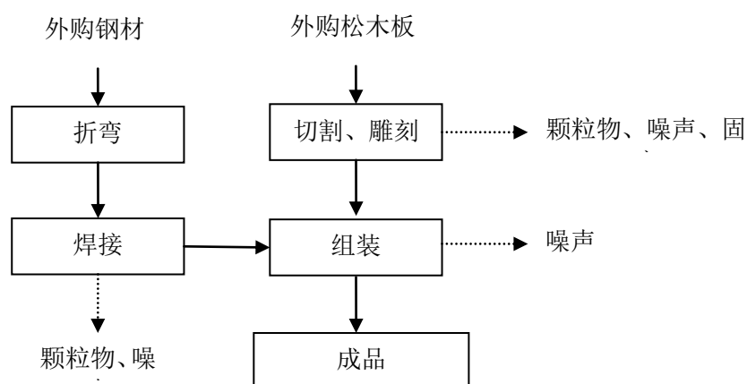
图一 项目工艺流程图
