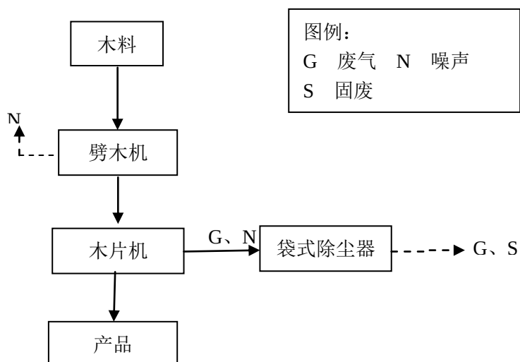
图一 生产工艺流程及产污环节示意图
