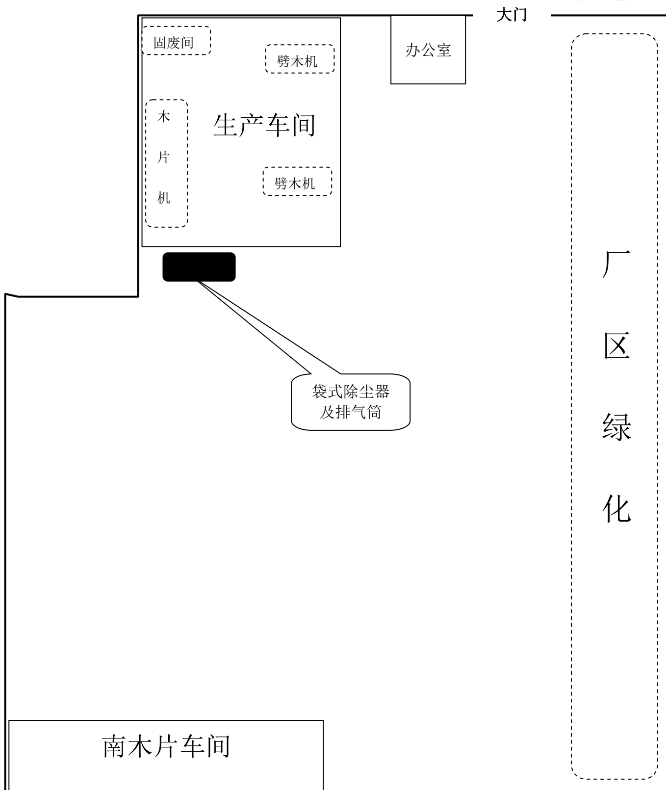
附图三 厂区平面布置图
