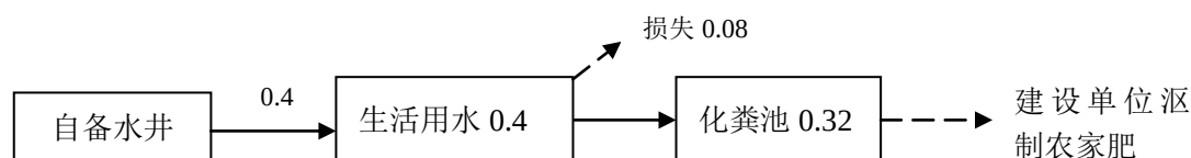
图二 本项目水量平衡图 ( \text{m}^3/\text{d} )
