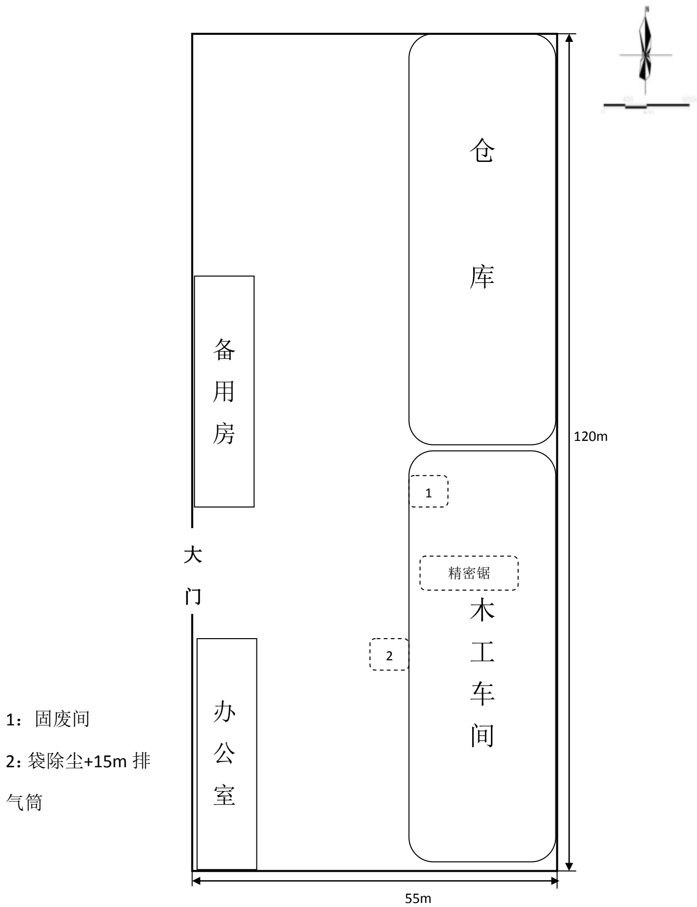
附图三 项目平面布置图
