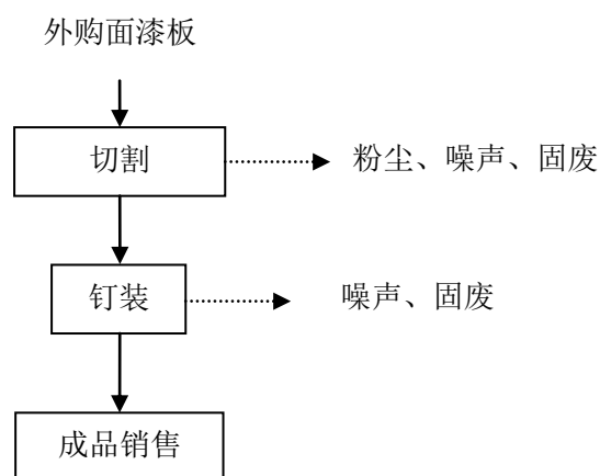
图一 项目工艺流程图
