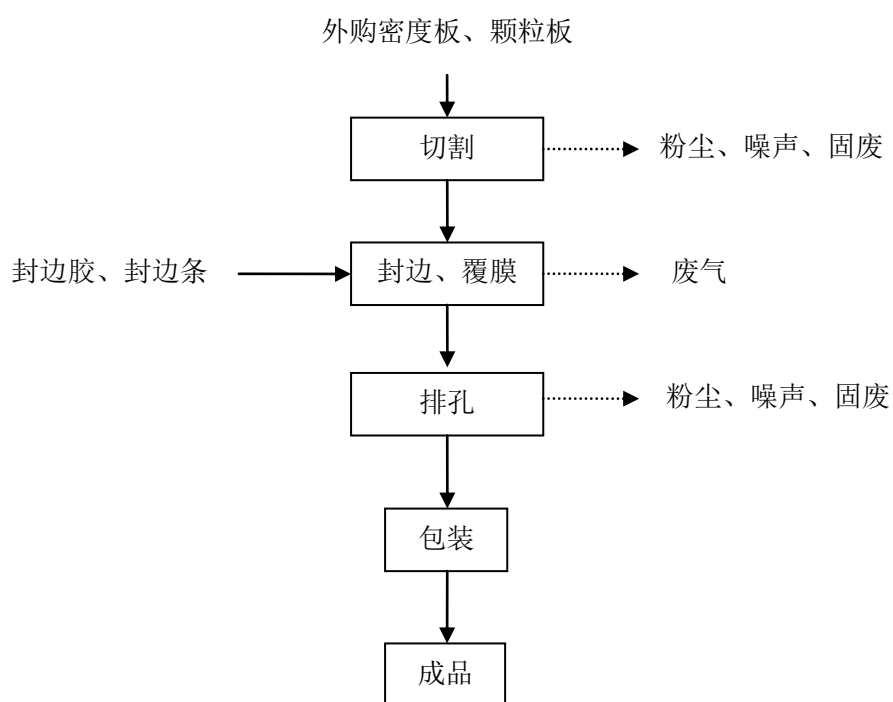
图一 项目工艺流程图
