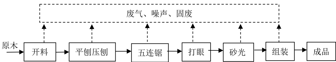
图 1 生产线工艺流程及产污环节图
