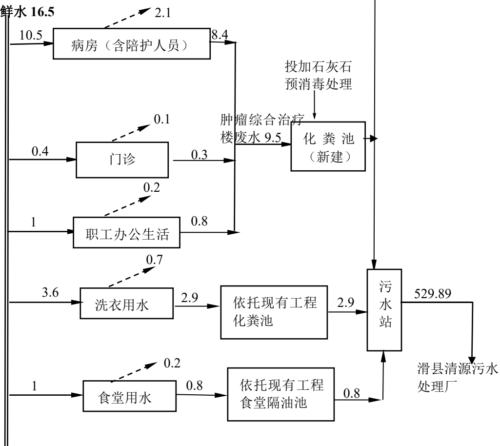
图 3 本项目建成后全院水平衡图（单位：m³/d）
