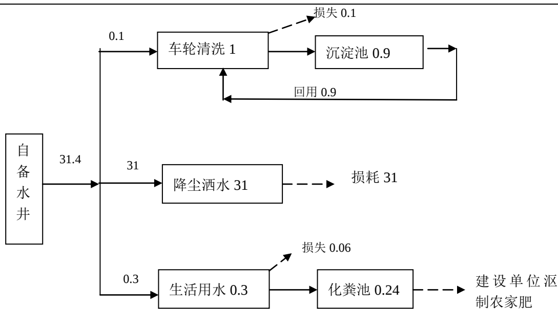
图三 本项目水量平衡图 (m³/d)
