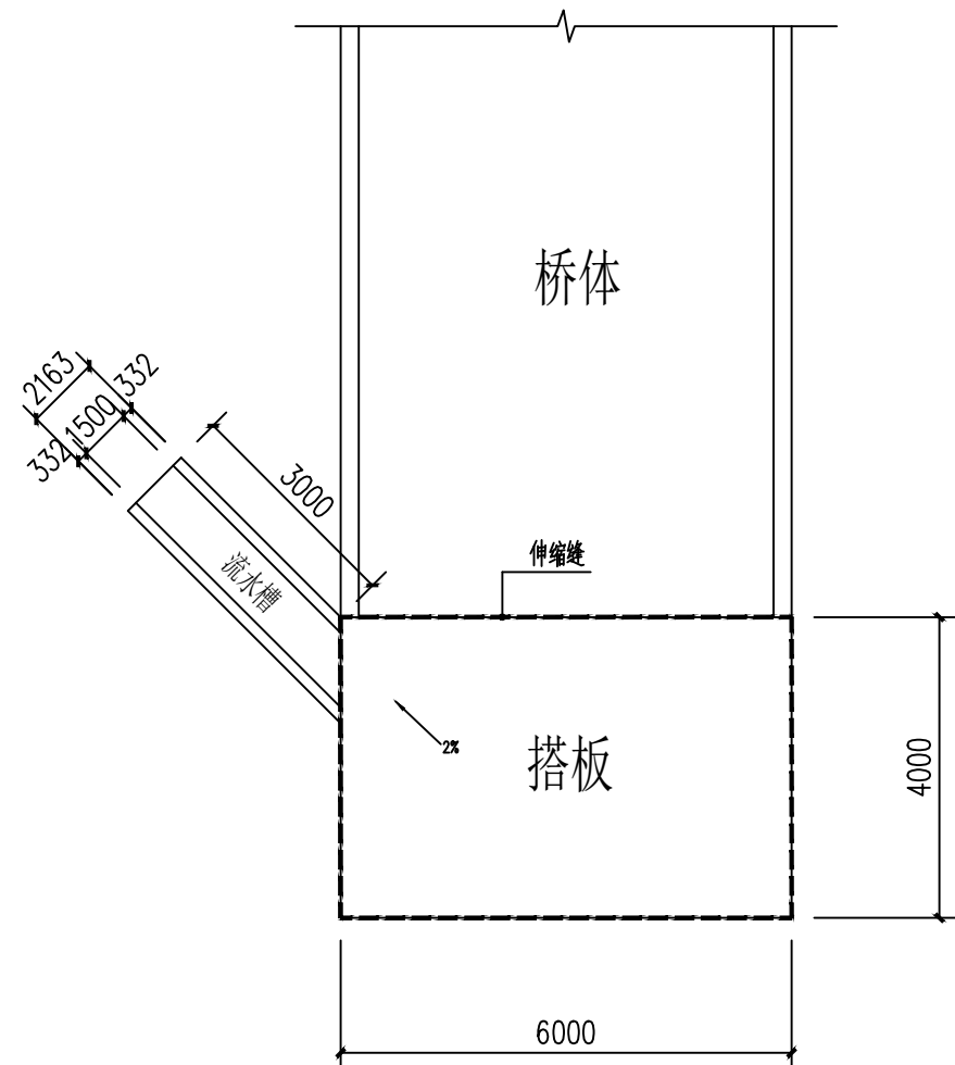
新建搭板平面图 1:100
