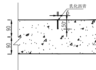
横向缩缝构造
