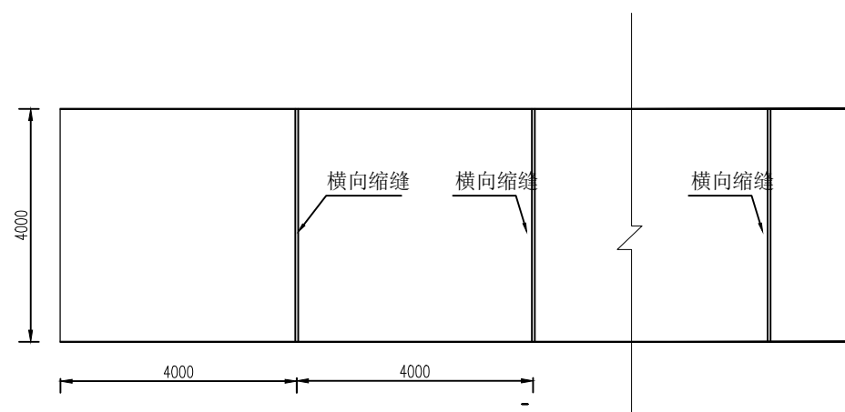
砼路面板横向缩缝分布图
