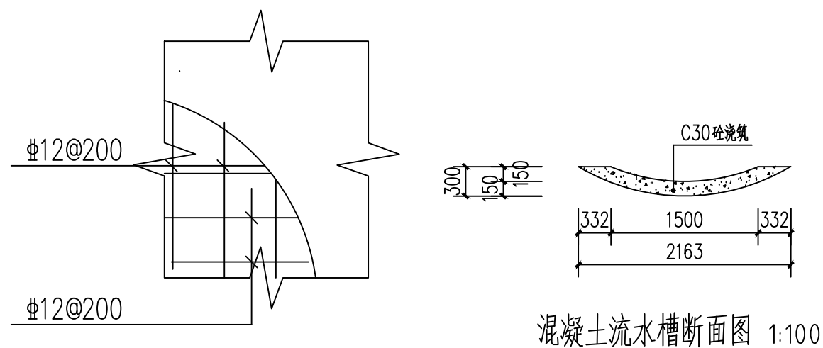
新建搭板配筋图 1:100
