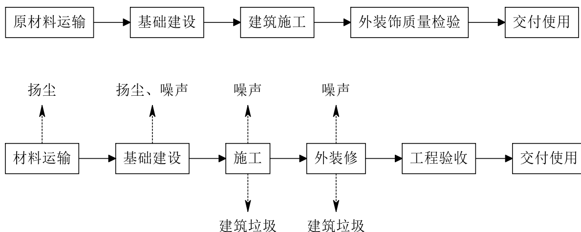
图一 污水厂施工期流程与产污环节图
